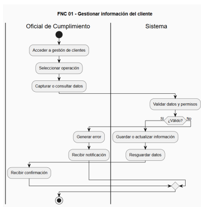
Figura 2. Detalles del Caso de Uso 01 y Diagrama de Actividades
